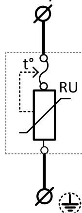
Рисунок 2. Электрическая схема добавочного УЗИП Комменж УЗФЭС-Д 75/15
