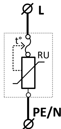
Рисунок 2. Функциональная схема подключения к электроустановке
